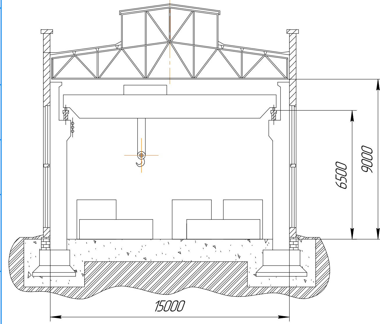
A-A (1:200)
